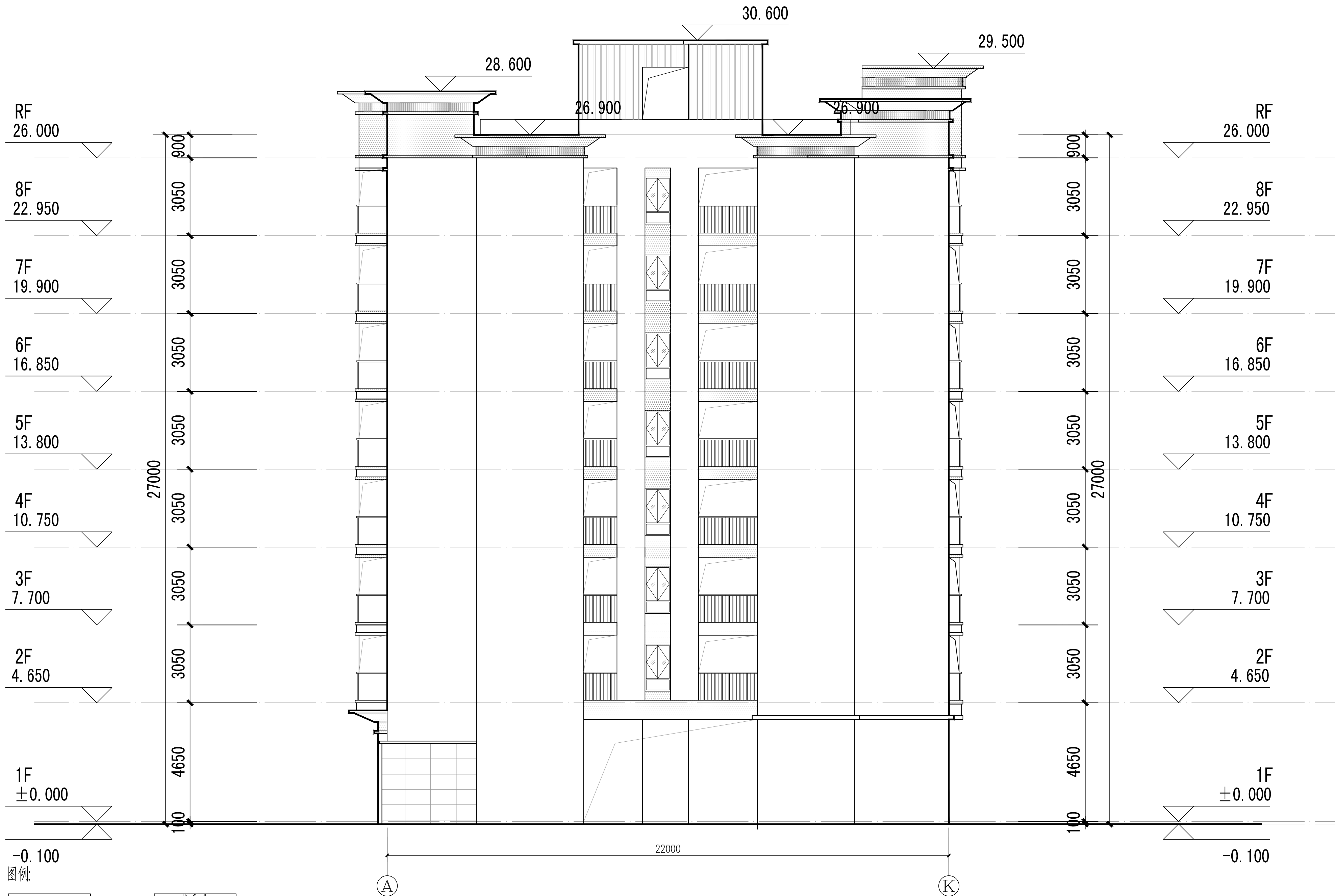
A-K 立面图 1:100
