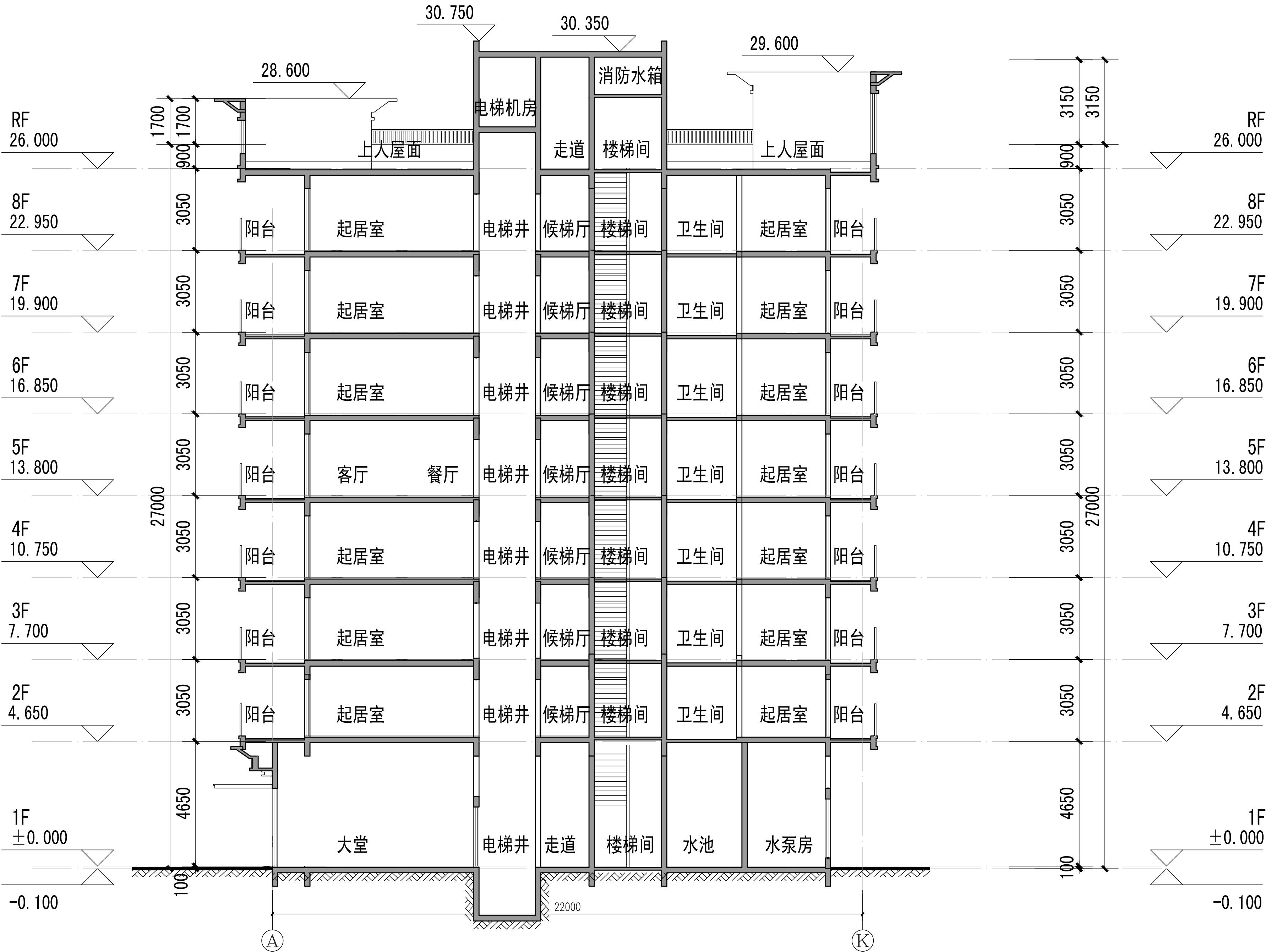
1-1剖面图 1:100
