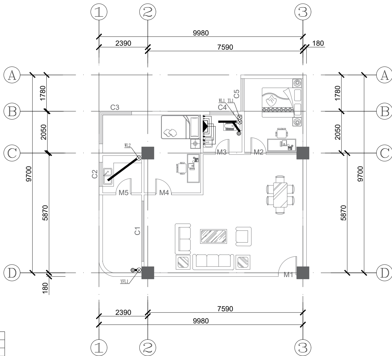
港口大厦A403给排水平面图
