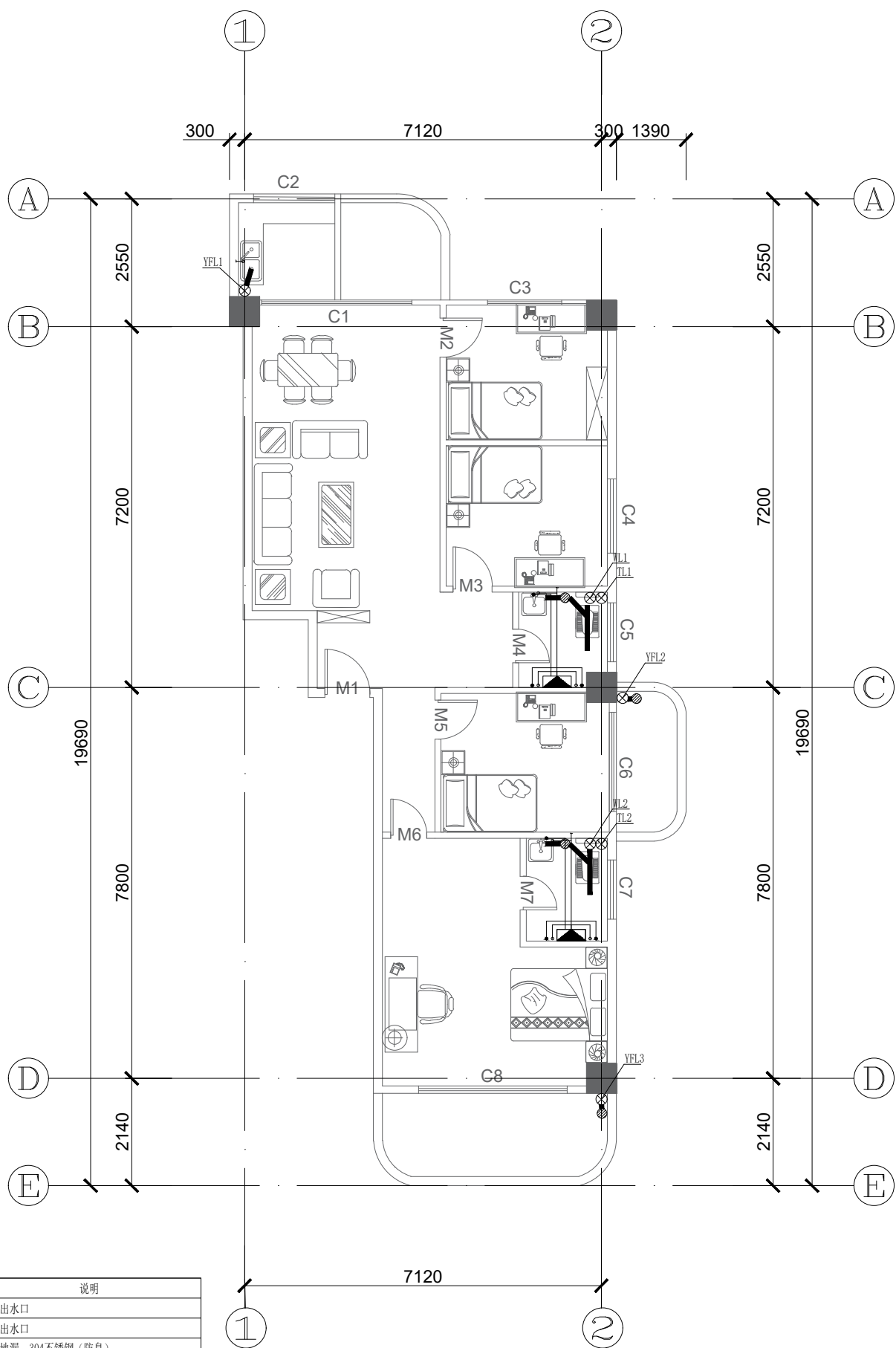
港口大厦A401给排水平面图
