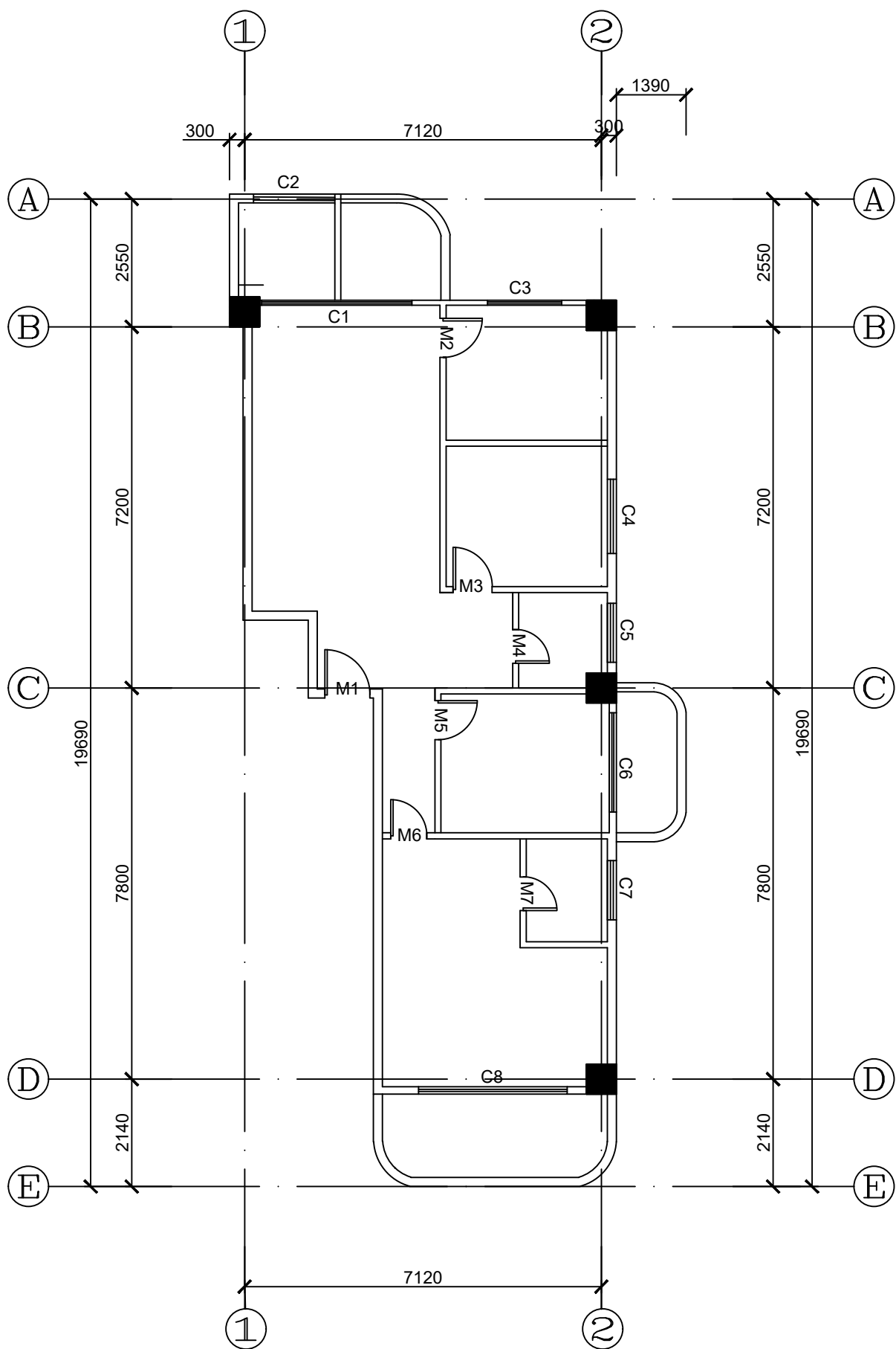
港口大厦A401平面图
