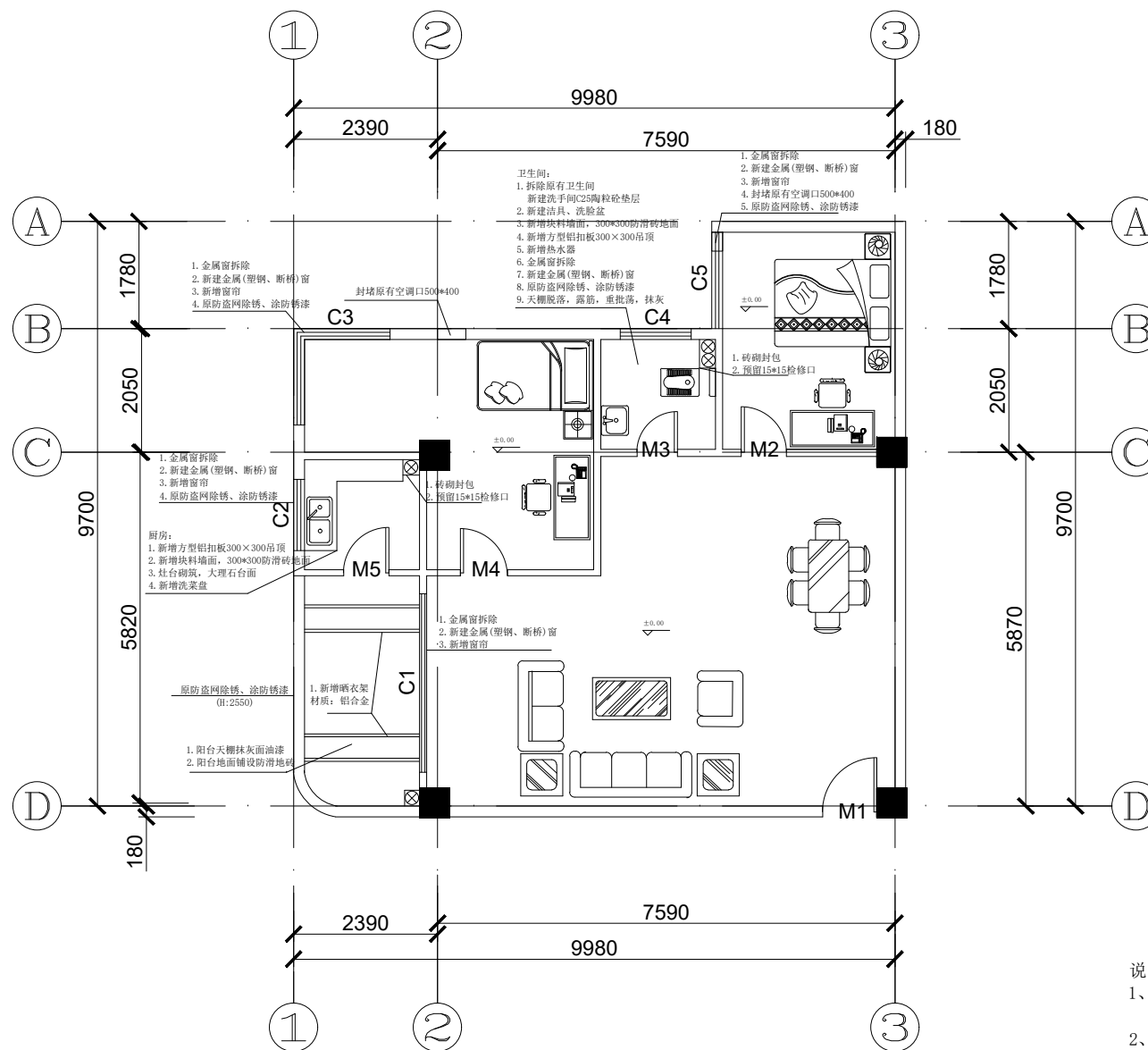
港口大厦A403平面布置图
