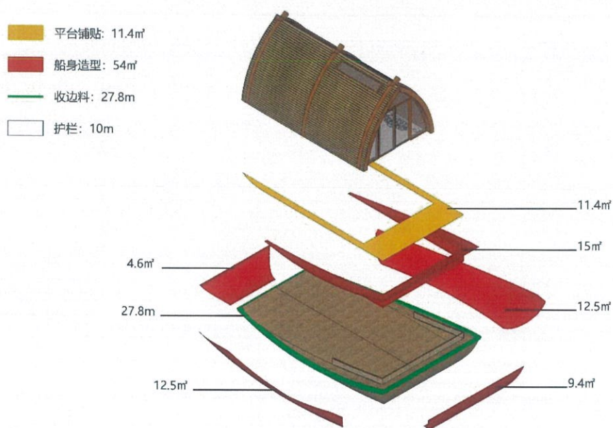
图 5 船屋室外空间铺贴分解示意
